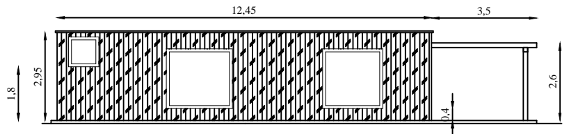
PROSPETTO D
