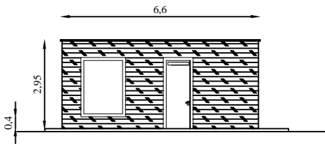
PROSPETTO C
